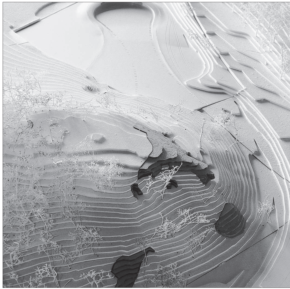
Der favorisierte Vorentwurf von Ritter Jockisch sieht eine Einbettung des halbrunden Archäopark-Besucherzentrums (im Bild oben) in die Landschaft am Vogelherd (unten) vor. Modellfoto: dam
